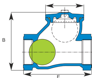
Gewindeanschluss
