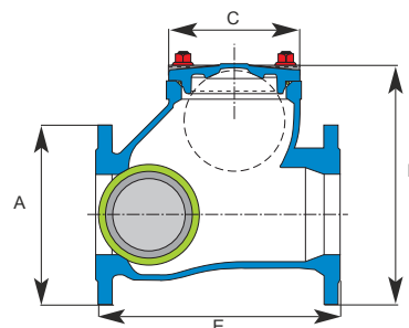
Flanschanschluss
